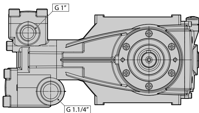
ГОЛОВКА MQ
