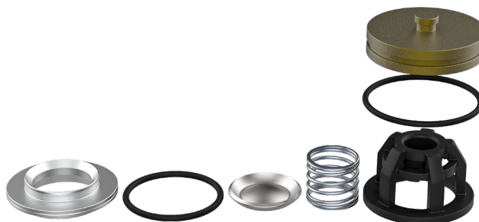
Питающий клапан для насосов с головкой MQ и HQ
