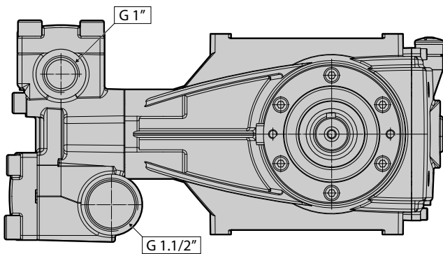
KOPF HQ
