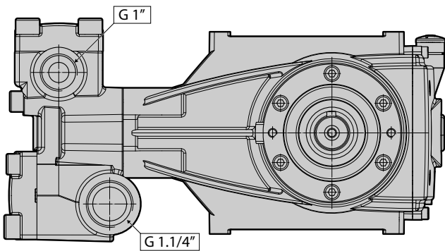
TÊTE LQ
