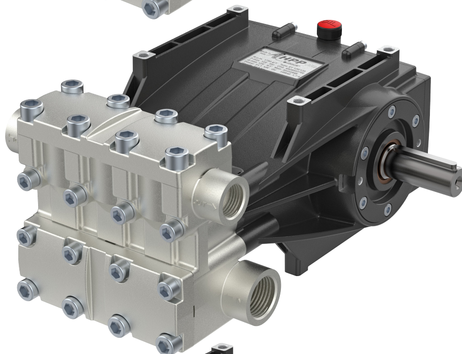
CABEÇOTE MQ
