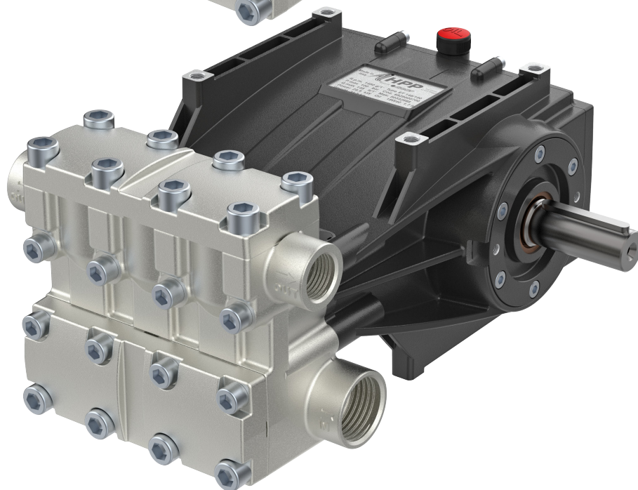
CABEZAL HQ
