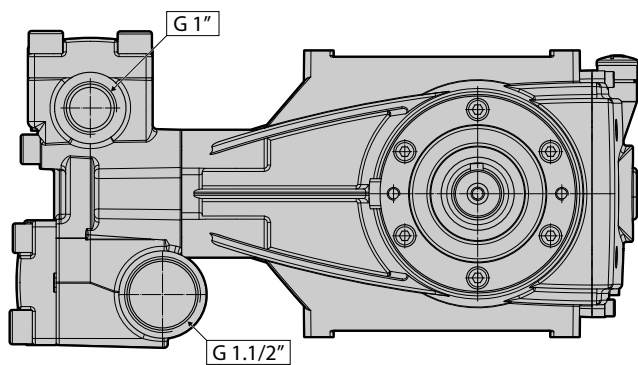
TÊTE HQ
