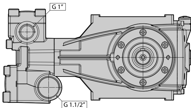
ГОЛОВКА HQ
