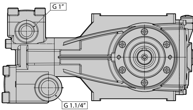
KOPF MQ
