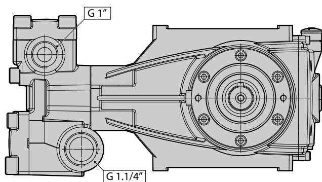
TESTATA LQ
