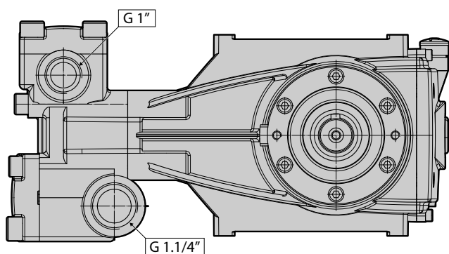
TESTATA MQ
