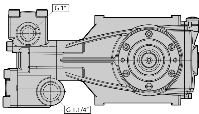
TÊTE MQ
